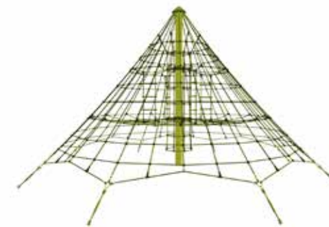
SEILNETZTURM II ROPE NET TOWER II 15.04.200 ⊕ Ø 8,00 m ⊕ Ø 10,00 m 📏 4,50 m 📏 1,50 m 😊 6+
