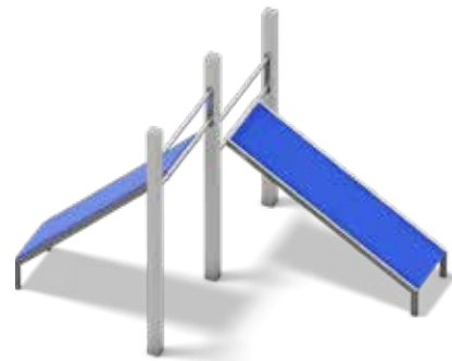
DOPPEL-BANK-SCHRÄG 30°/ 45° DOUBLE BENCH 30° / 45° 12.06.171 ⊕ 2,30 x 2,47 m ⊕ 5,30 x 5,48 m ⊕ 1,66 m
