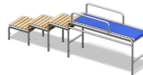
SQUAT-PLATTFORM UNIVERSAL SQUAT-PLATFORM UNIVERSAL 12.06.173 ⊕ 3,74 x 0,69 x 1,28 m ⊕ 6,74 x 3,69 m ⊕ 0,99 m
