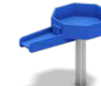
VERTEILER, DREHBAR FEEDING BASIN, TURNABLE 11.14.292 ⊕ Ø 1,37 m
