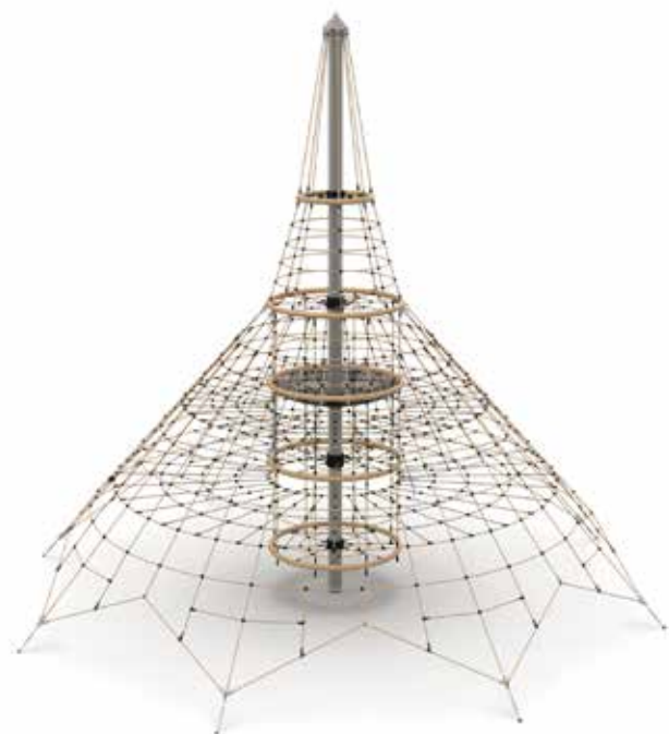
SEILNETZ-PYRAMIDE DINO XXL ROPE NET PYRAMIDS DINO XXL 15.04.101 Pyramide Dino XXL ⊕ Ø 9,55 m ⊕ Ø 11,00 m 📏 8,20 m 📏 1,75 m 😊 4+
